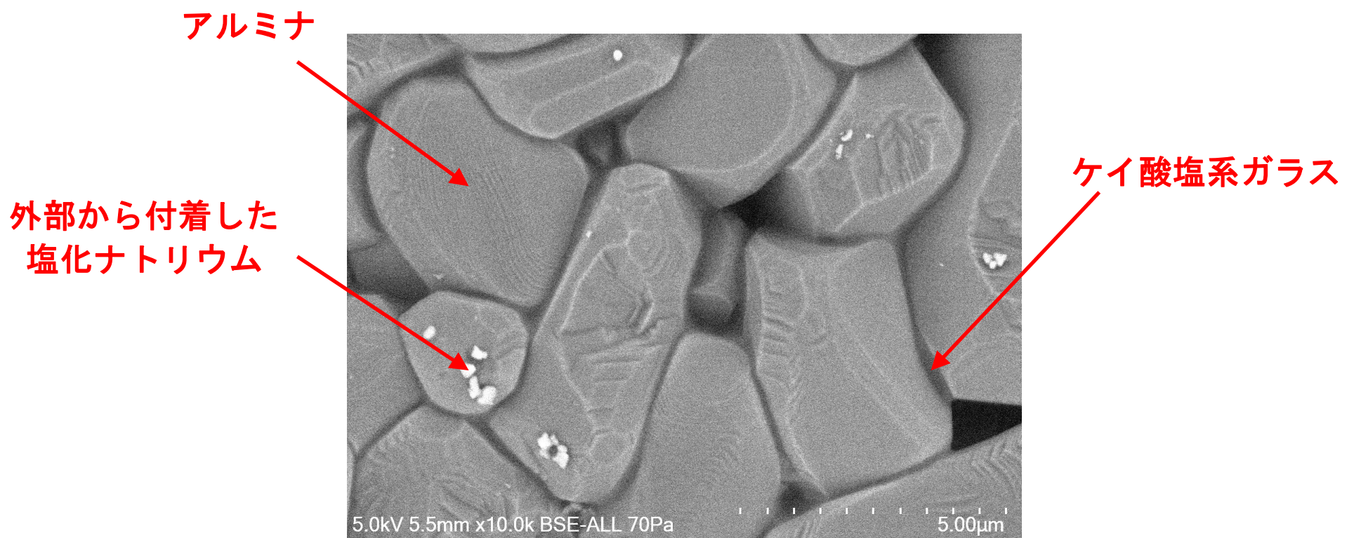
反射電子組成像 ×10,000
