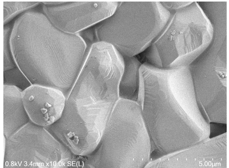
二次電子像 ×10,000
