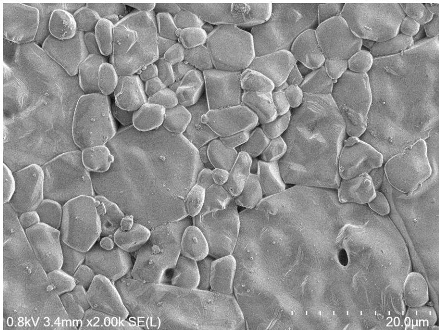
二次電子像 ×2,000
